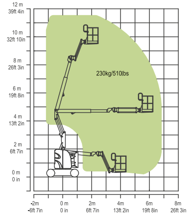
ZA10RJE Çalışma Diyagramı
