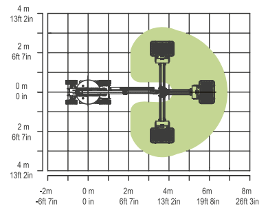
Jib Bom Döndürme Hareketi – ZA10RJE
