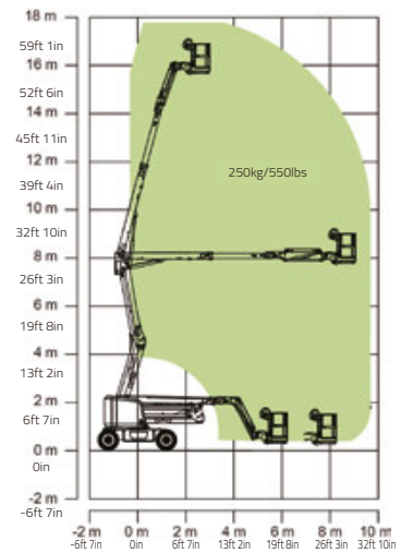
Hareket Aralığı ZA16JERT/ZA16JERT-Li
