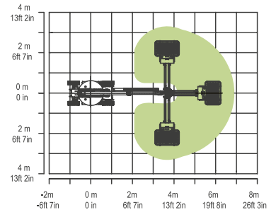
Jib Bom Döndürme Hareketi – ZA10RJE
